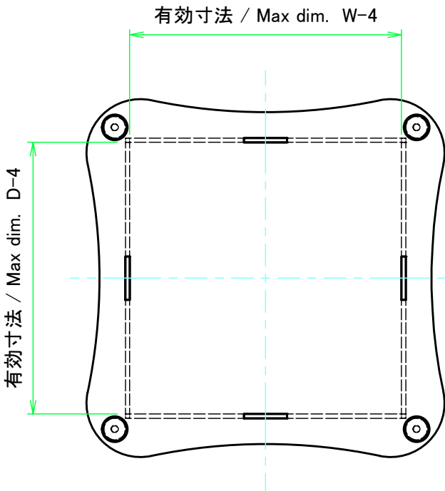
下カバー / Bottom cover
