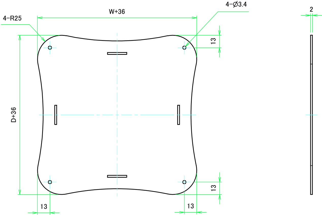
上カバー表面 / Top cover Frontside
